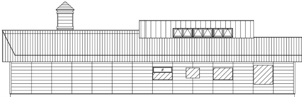
改修後 北立面図
