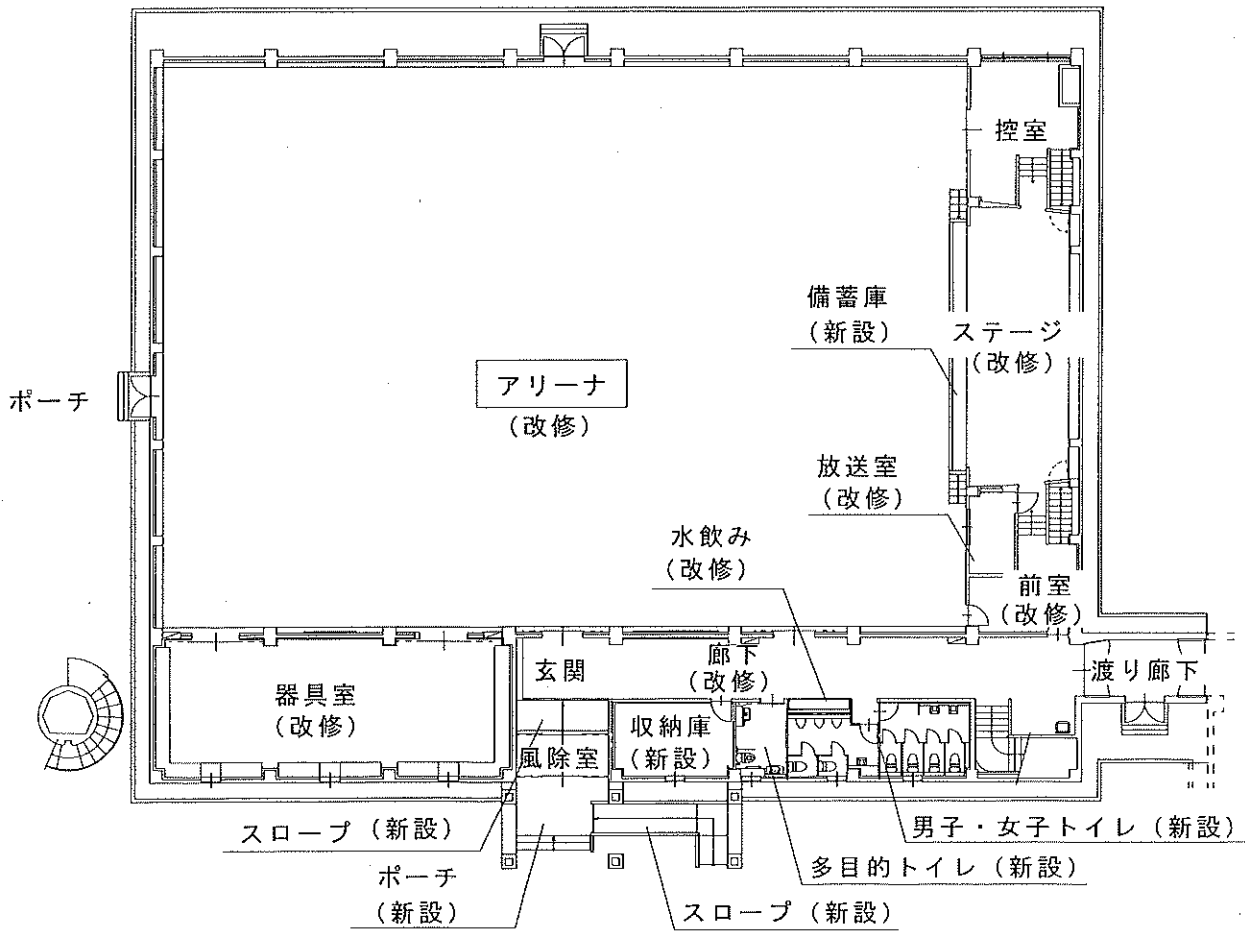
1階平面図 (改修後)
