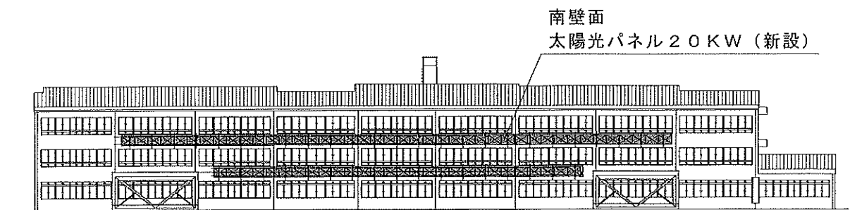
南側立面図
