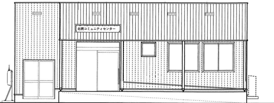
南立面図
