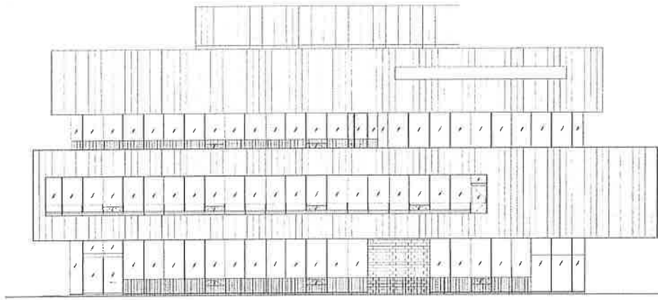
南立面图
