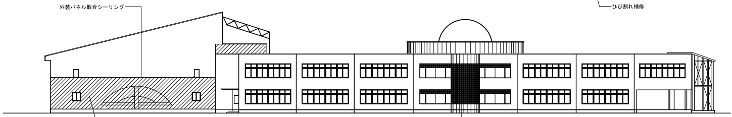
南側立面図
