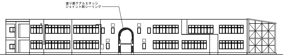
南側立面図
