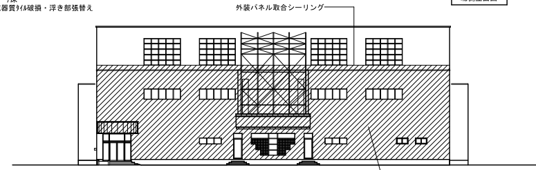
東側立面図
