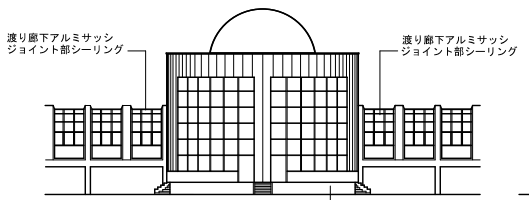
西側立面図
