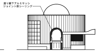
北側立面図
