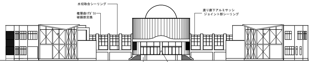
東側立面図
