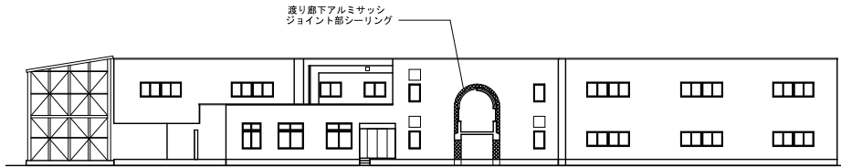
北側立面図
