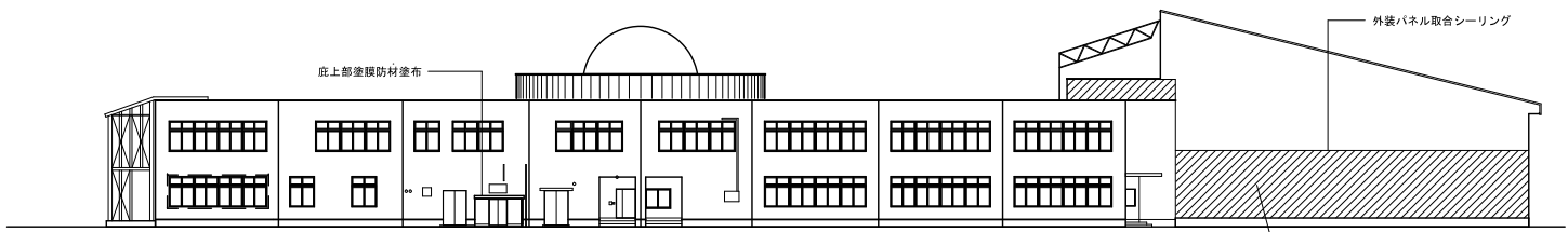
北側立面図
