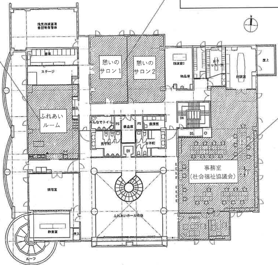
2階平面図
