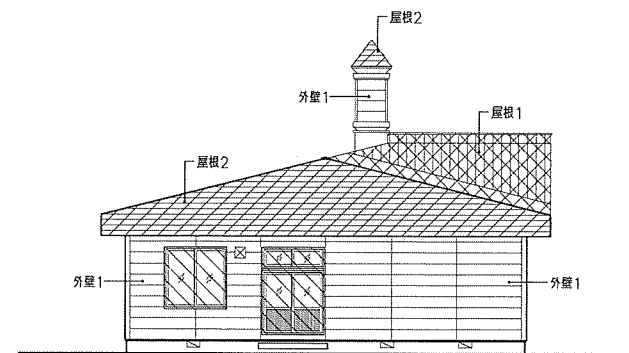
改修前 西立面図
