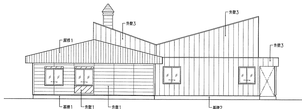
改修後 西立面図
