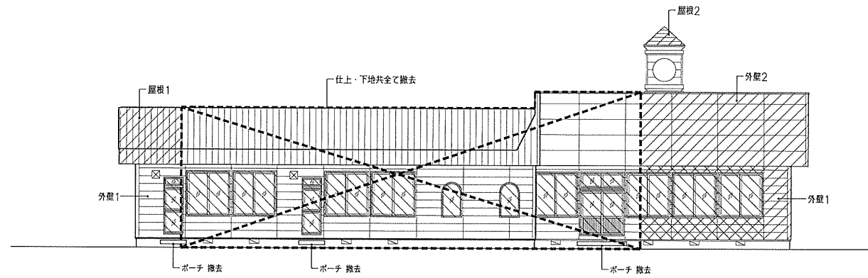
改修前 南立面図
