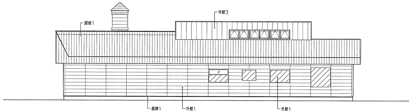
改修後 北立面図
