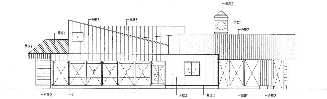
改修後 南立面図
