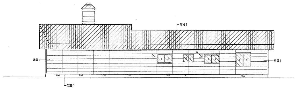
改修前 北立面図
