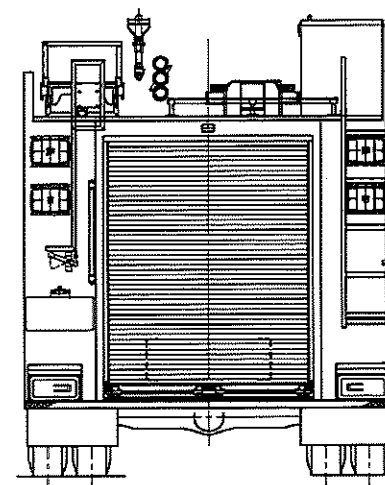
幕別消防署 水槽付消防ポンプ自動車 構想図
