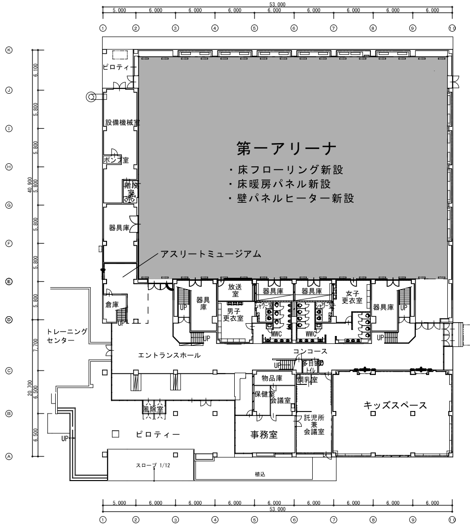
平面図（1階）
