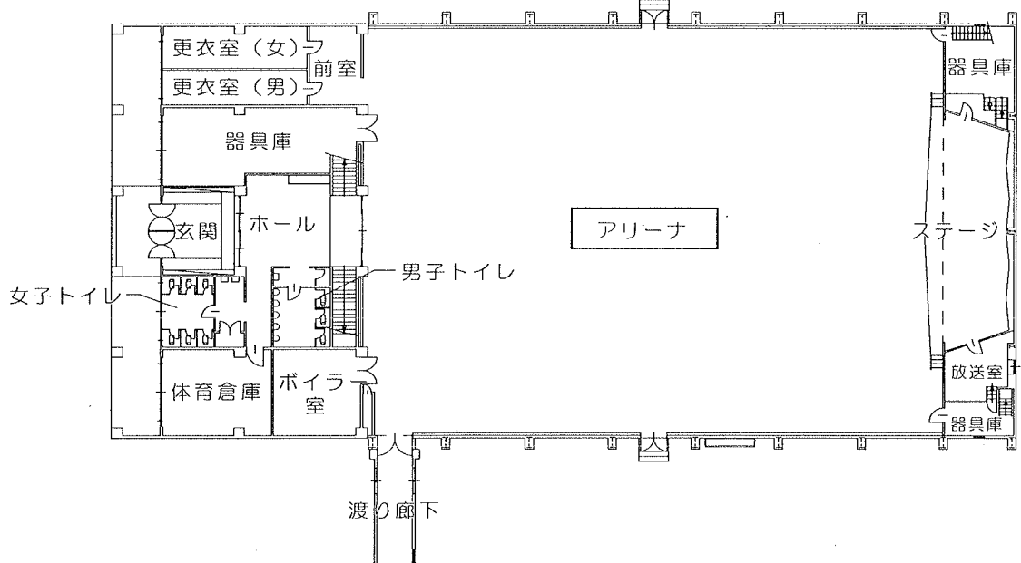
1階平面図 (改修前)
