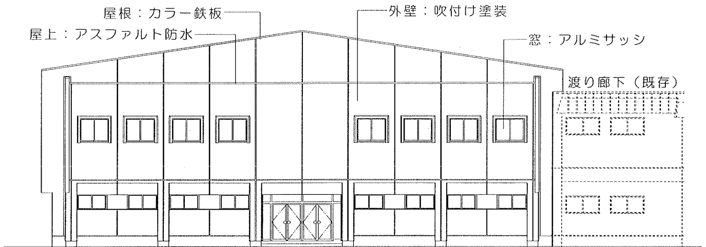
南側立面図（改修前）
