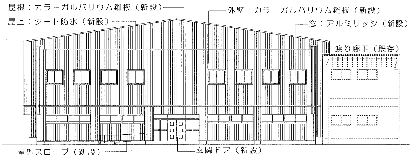
南側立面図（改修後）
