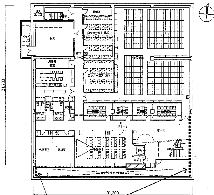
B1階平面図
