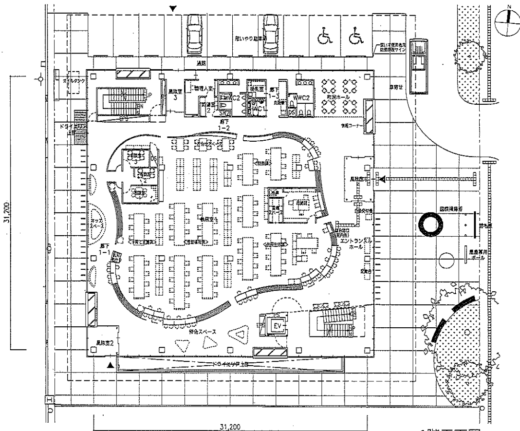
1階平面図
