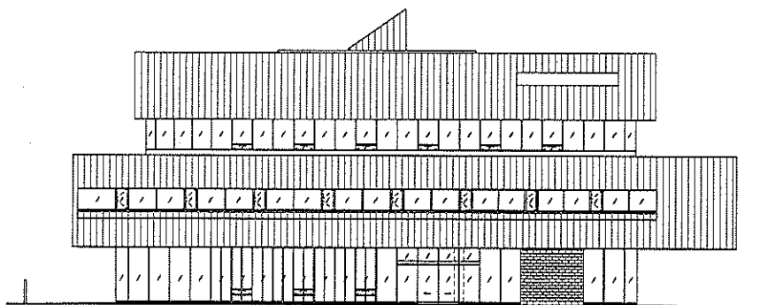
東立面图
