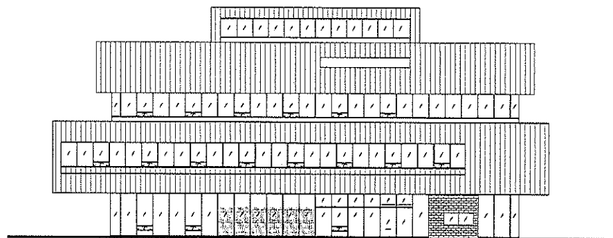
北立面图
