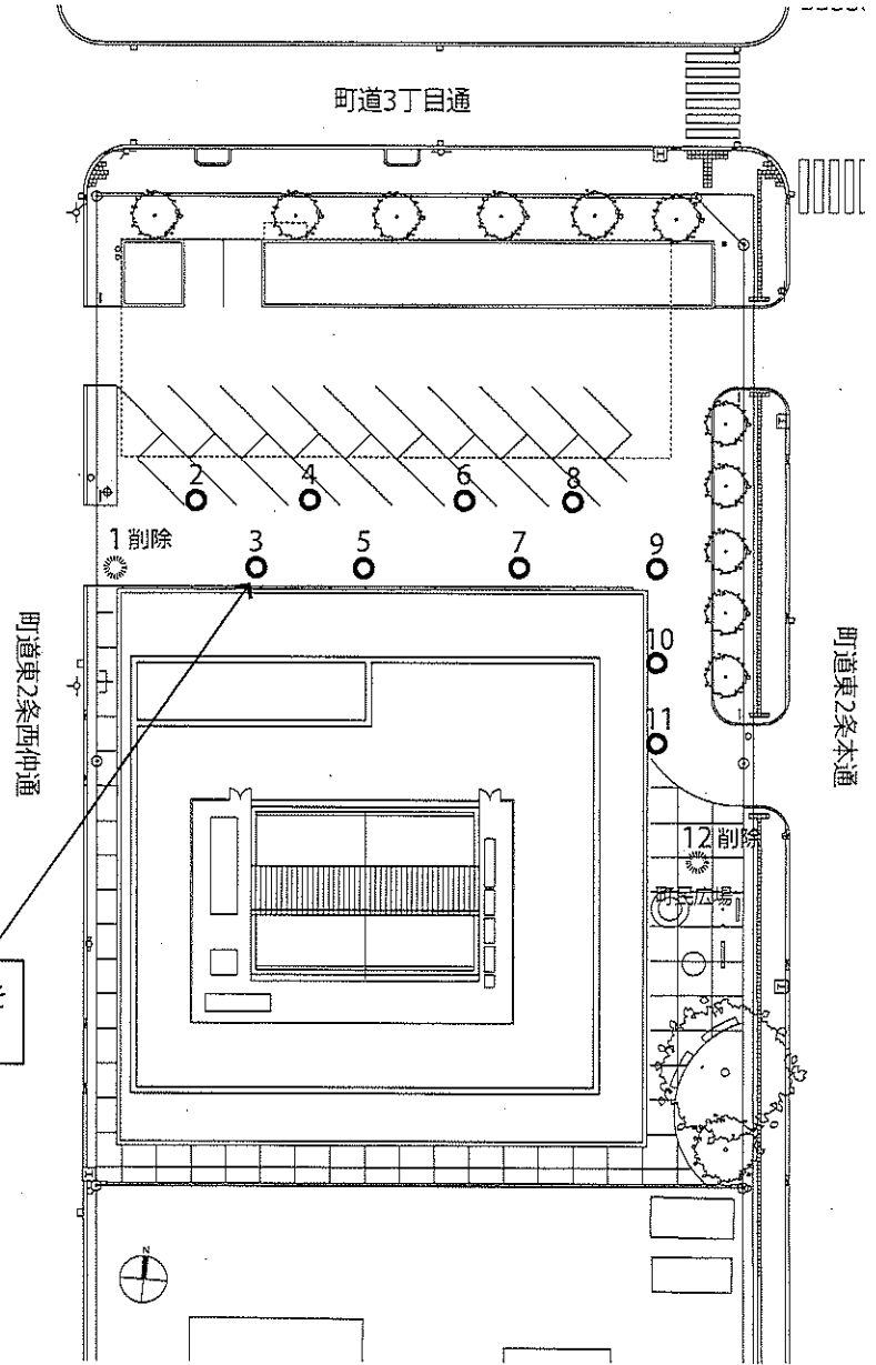
配置図
