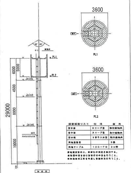
無線柱構造図
